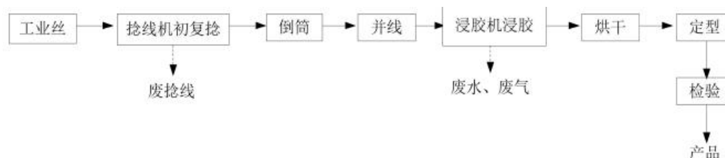
图 4.1.3-7 工程用浸胶硬、软线绳生产工艺流程图
