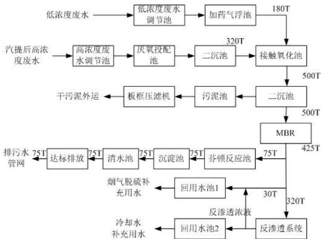
图 4.1.4-2 污水处理站工艺流程图
