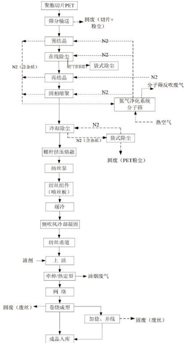
图 4.1.3-4 差别化涤纶工业丝生产工艺流程图
