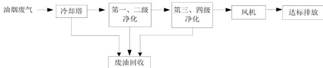
图 4.1.4-1 静电除油装置处理工艺流程图
