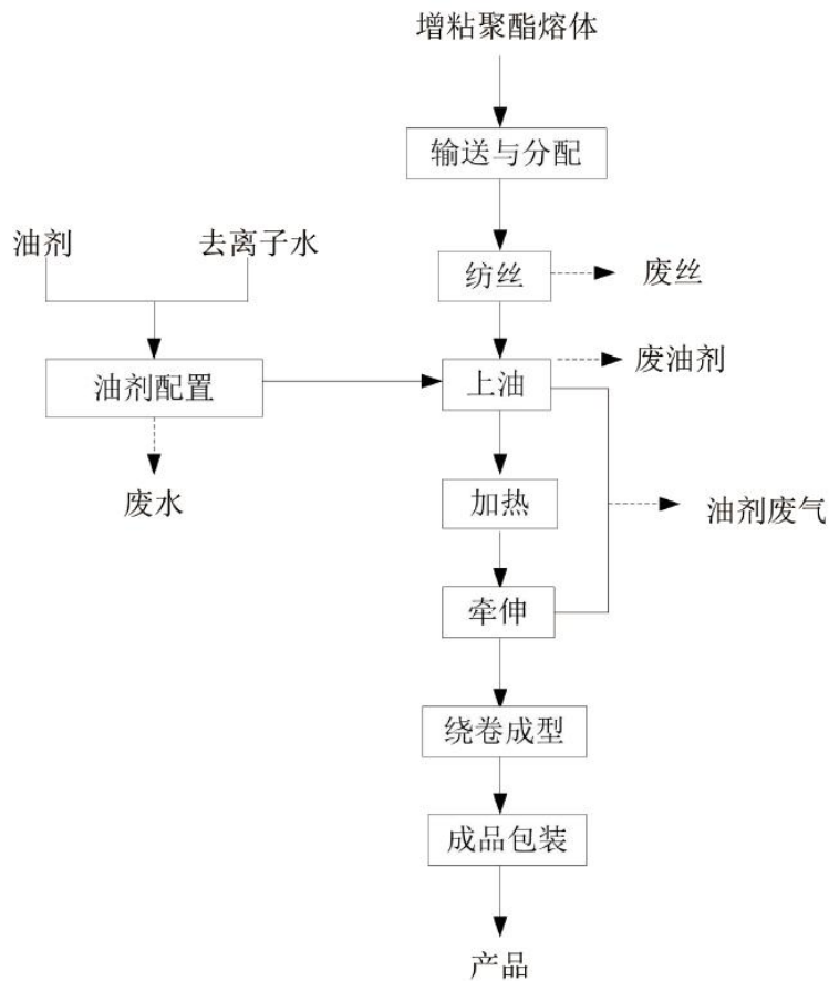
图 4.1.3-8 直纺差别化工业丝工艺流程图
