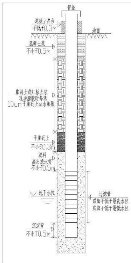
图 7.4-1 地下水监测井结构示意图
