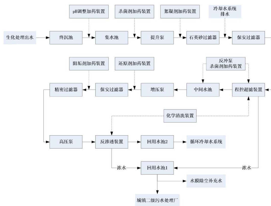
图 4.1.4-3 中水回用深度处理工艺流程图
