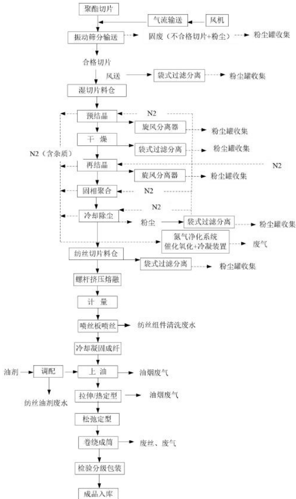
图 4.1.3-9 高端工业丝生产工艺流程及产污节点图
