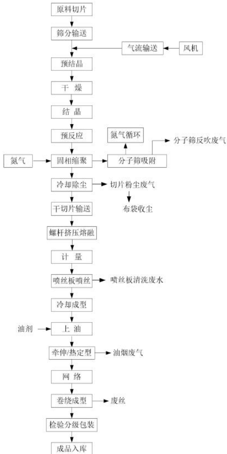
图 4.1.3-1 涤纶工业丝工艺流程及产污环节示意图
