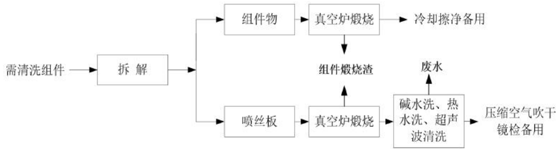
图 4.1.3-10 纺丝组件清洗工艺流程图
